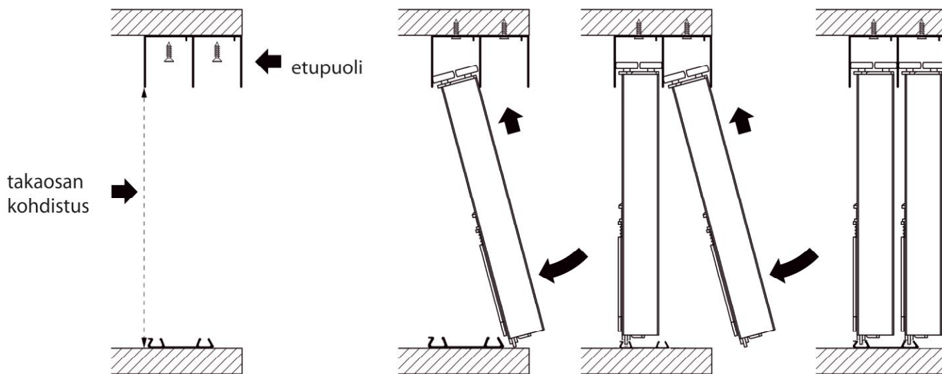
6 kiskojen sijoittaminen
