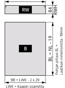
Takasaran ja pohjalevyn mitoitus Materiaalipaksuus 16mm
