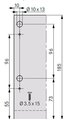
Takasarjan asennusmitat
