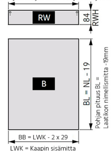
Takasarjan ja pohjalevyn mitoitus Materiaalipaksuus 16mm
