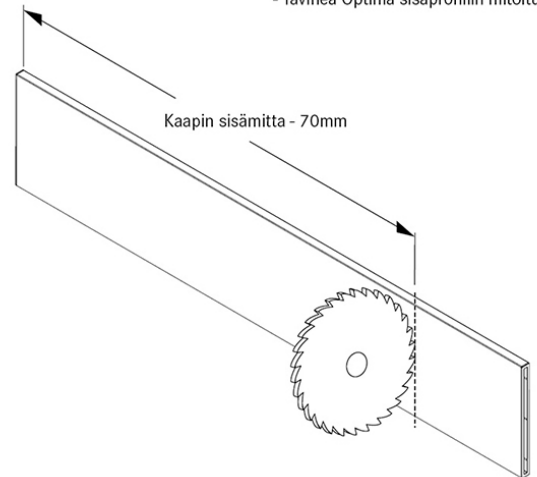
Nova Pro Scala - Tavinea Optima sisäprofiilin mitoitus
